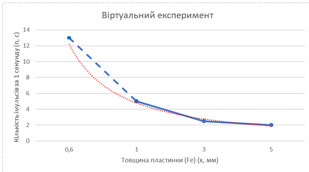
Рис. 4. Графік залежності: n(c) – кількості імпульсів, обрахованих ОПЗ на Python 3.9, x(мм) – товщини залізної (Fe) пластини, за результатами віртуального дослідження «Визначення коефіцієнта поглинання \gamma -випромінювання»
